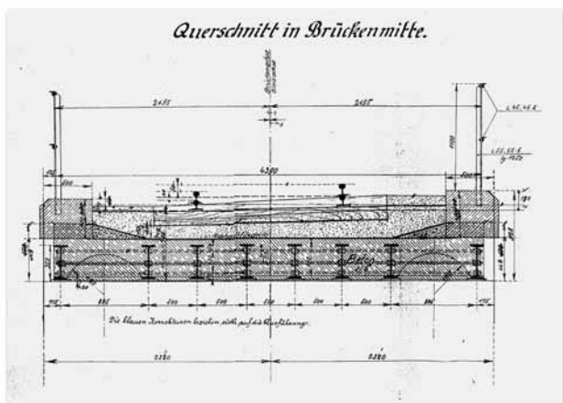
Příčný řez mostkem z technické dokumentace
